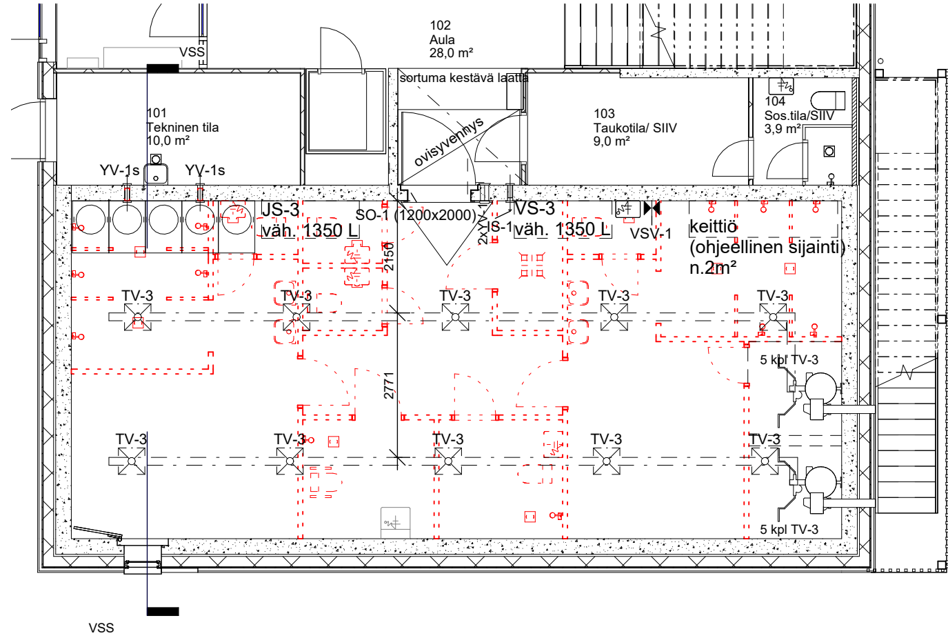
1.krs VSS 1 : 100
