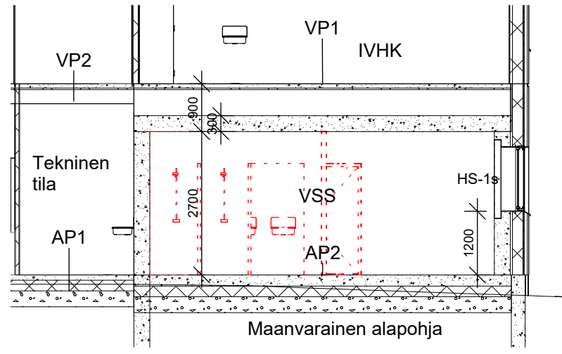
VSS 1 : 100
