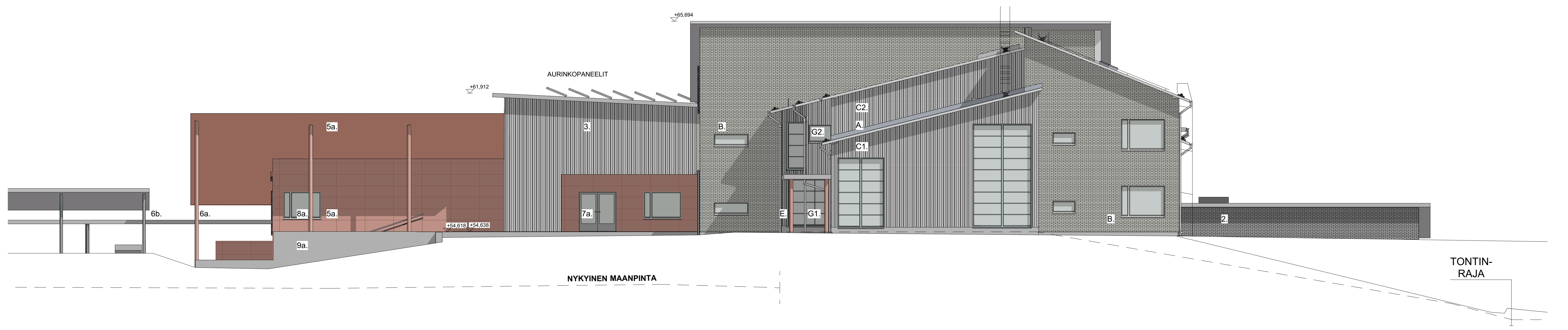
Julkisivu kaakko
